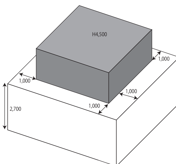
【立面】
