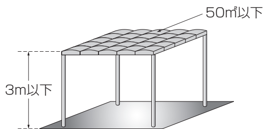
図A 防災設備等の感知及び散水障害とならない場合
