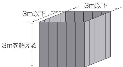
図A 防災設備等の感知及び散水障害とならない場合
